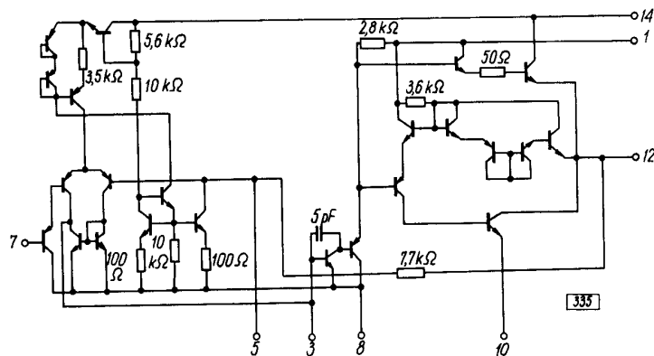
Schemat elektryczny
